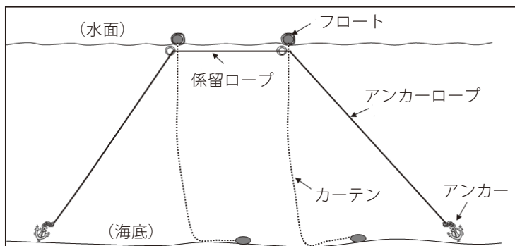
◀シルトフェンスの断面イメージ図
